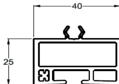
Verbreiding rolluikgeleider
