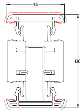
Vertikaal koppelprofiel
