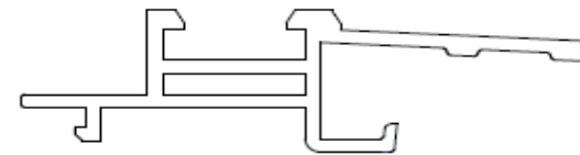
Speciale groef (naast raamkader tot 10 mm)
