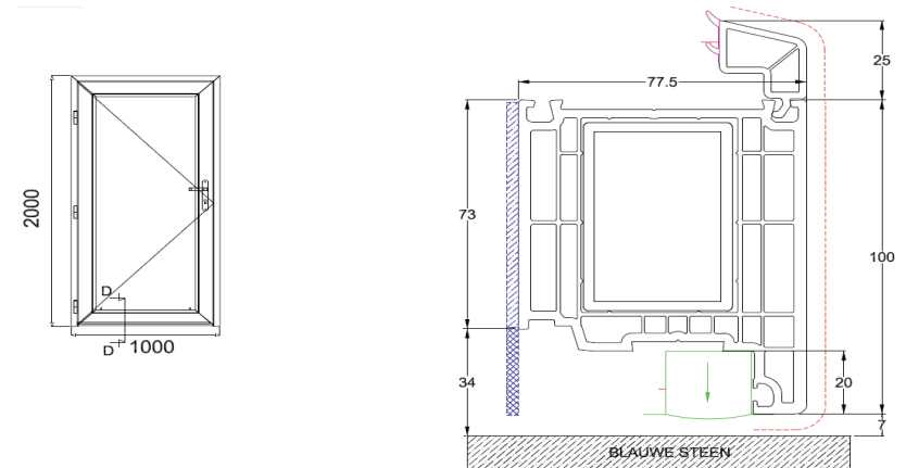
ThermoSense Doorsnede D/D
