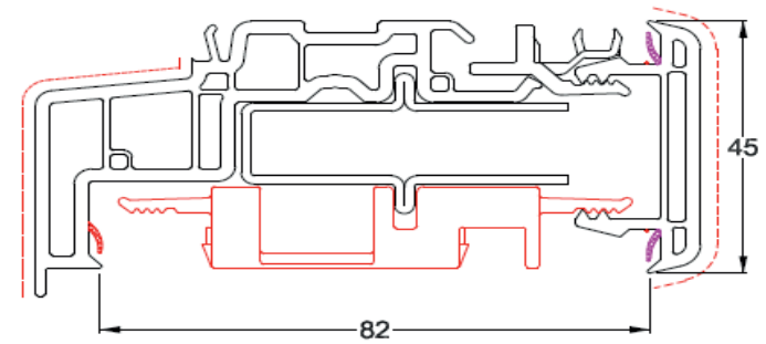
Horizontaal koppelprofiel
