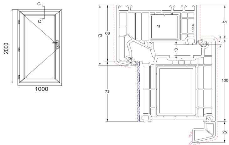
ThermoSense Doorsnede C/C
