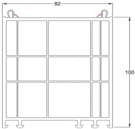
Verbreidingsprofiel 100 mm.
