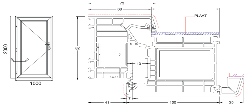
ThermoSense Doorsnede A/A
