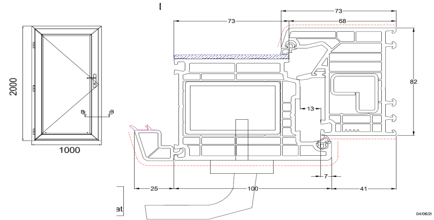
ThermoSense Doorsnede B/B
