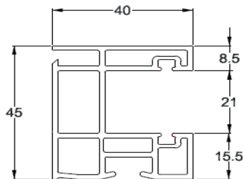
Rolluikgeleider
