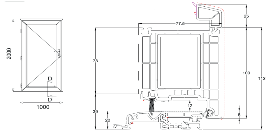
ThermoSense Doornsnede D/D onderdorpel
