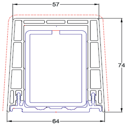
Versterking voor Traverse
